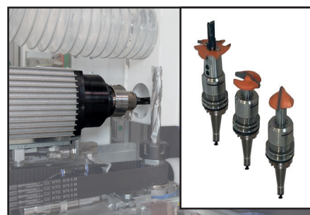
Fresador con cono ISO intercambiable: incluye 4 conos ( 1 con motor + 3 sin herramienta).
