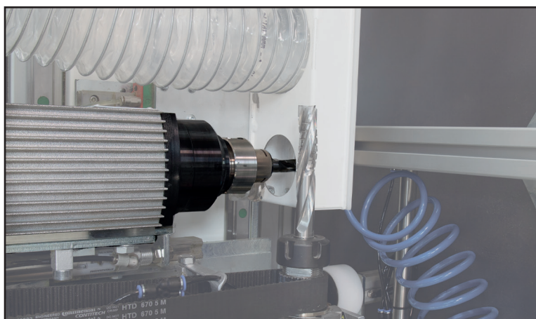
Motor fresador que realiza fresados frontales, orificios de maneta, abertura de vidrieras y ranurados decorativos.
