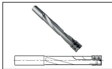
Fresa para cerraduras con inserto intercambiables.
