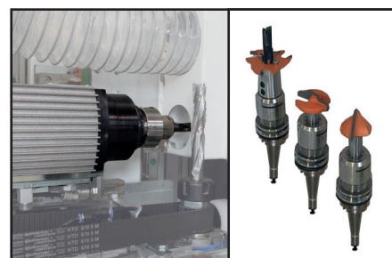
Fresador con cono ISO intercambiable: incluye 4 conos ( 1 con motor + 3 sin herramienta).
