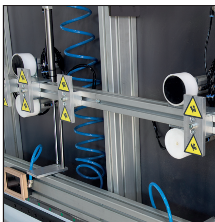
Mesa adicional para mecanizado de marcos.
