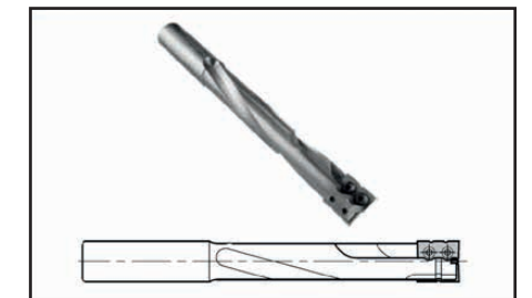
Fresa para cerraduras con inserto intercambiables.
